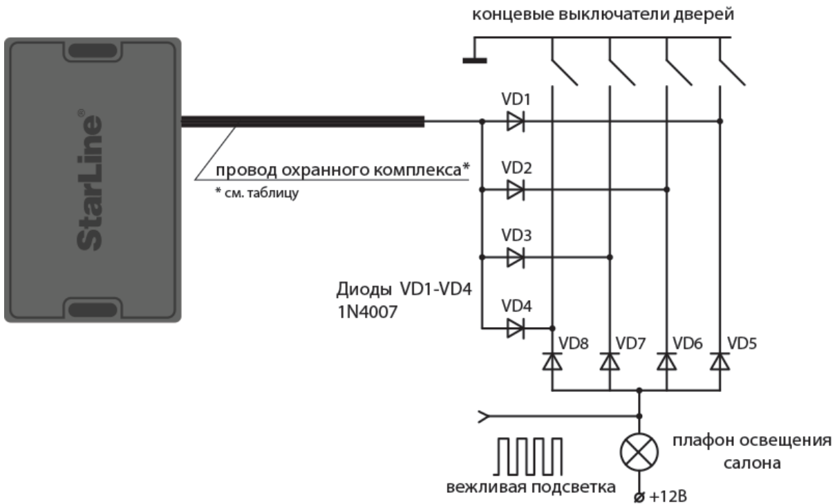
Схема светодiodeйной развязки для концевых выключателей отрицательной полярности
